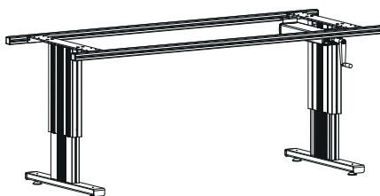
ERGO-Flex, Grundgestell mit Handkurbel höhenverstellbar mit Handkurbel von 720 – 1020 mm, Flächenbelastung 350 kg
