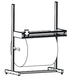
Einfach-Schneidgerät, stationär hoch für individuellen Aufbau mit Zubehör ab Seite 66, mit 1 Schneidrahmen, Achsaufnahme und Achse für Rollendurchmesser 750 mm
