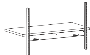
Kabelkanal zwischen Säulen Nutzhöhe 70 mm, für Steckdosenleiste (siehe Seite 93)
