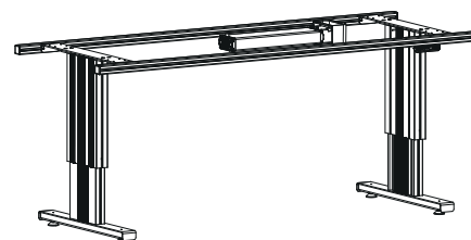
ERGO-Flex, Grundgestell mit Elektromotor höhenverstellbar mit Elektromotor von 720 – 1120 mm, Flächenbelastung 400 kg
