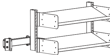
Typ 4 komplett inkl. 2 Ablageböden mit verschraubten Konsolen 660 x 270 mm
