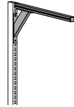
Ausleger komplett inkl. 30/30 Aluprofil Länge 670 mm
