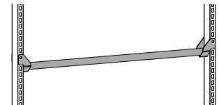
Achsauflage zwischen Lochprofilen bestehend aus 1 Satz Achsauflagen und 1 Achse Ø 33 mm
