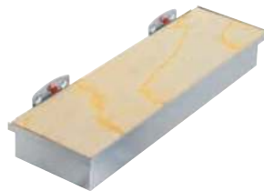
Werkzeugaufnahmebox mit Holzplatte zum Selbstbohren, Aufnahme: 320 x 135 x 55 mm, alufarben
